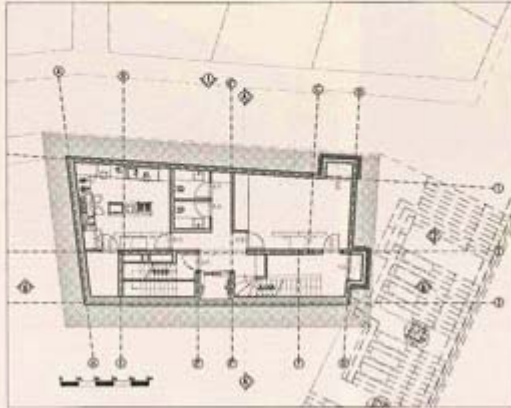
İkinci Bodrum Katı Planı Second Basement Floor Plan
