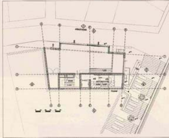
Zemin Katı Planı Ground Floor Plan
