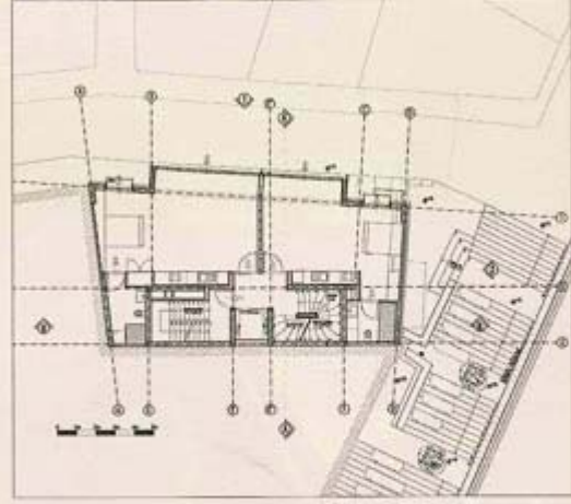
1-6. Kat Planları 1-6th Floors Plan
