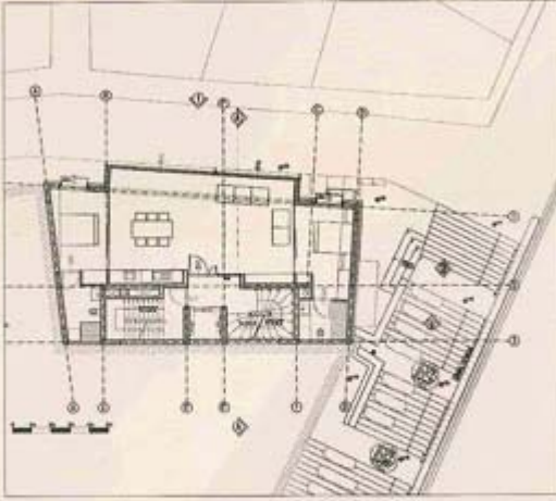
Yedinci Kat Planı 7th Floor Plan
